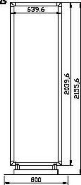
Vorderansicht M 1:25
