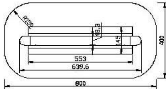
Vorderansicht M 1:25
